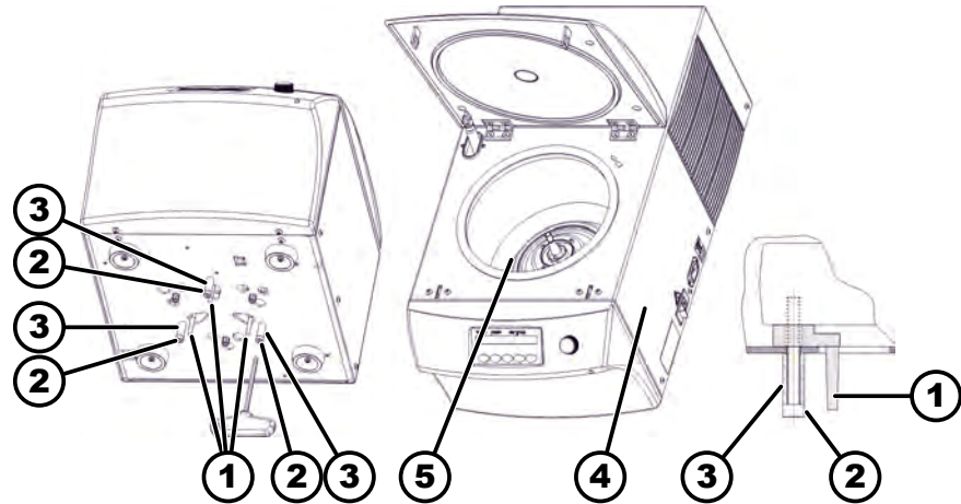
Abb. 13: Transportsicherung
