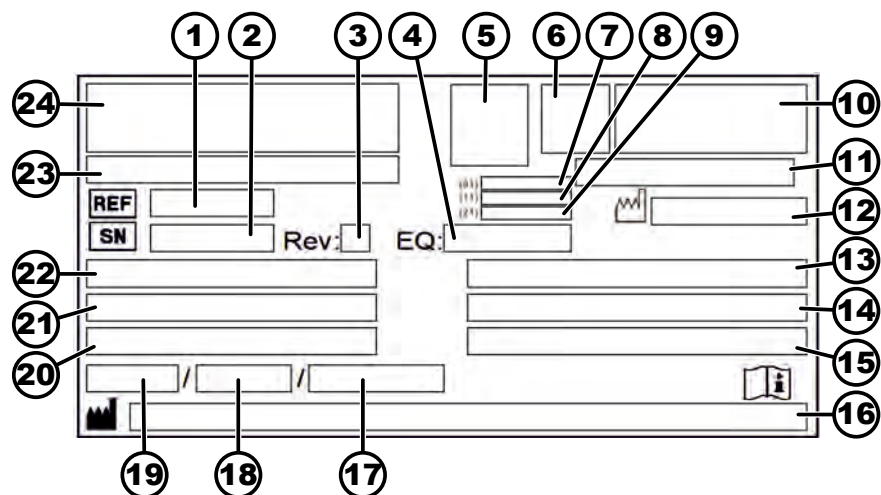
Fig. 1 : Plaquette signalétique
