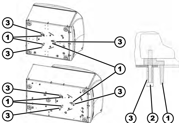
Abb. 14: Transportsicherung
