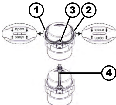
Abb. 20: BIO-Sicherheitssystem
