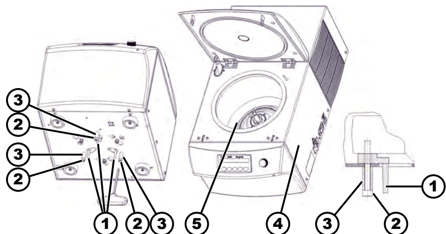
Abb. 14: Transportsicherung
