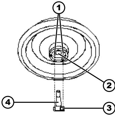
Abb. 15: Ein-Ausbau Rotor
